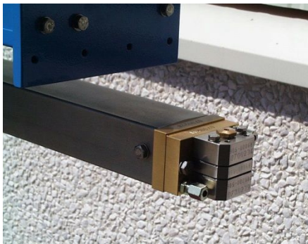
GSK-P mit Standardsprühkopf für Einzel-Gesenkstation
