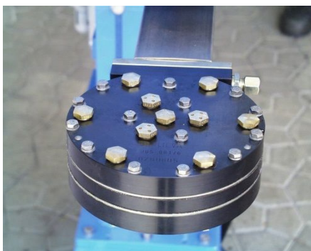
GSK-P mit Sondersprühkopf für rotationssymmetrische Teile
