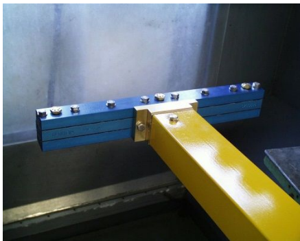
GSK-P mit Sondersprühkopf für drei Gesenkstationen
